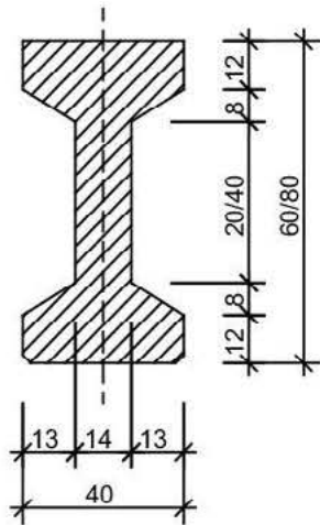
PRZEKRÓJ A-A
