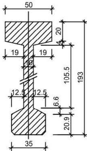
PRZEKRÓJ A-A TYP 2
