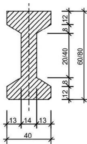
PRZEKRÓJ B-B
